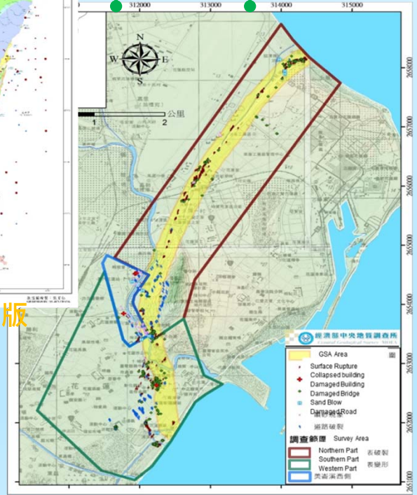
米崙活動斷層地質敏感區(105公告)
