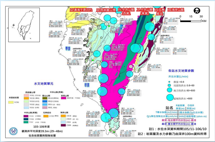
山區場址供水潛能圖
