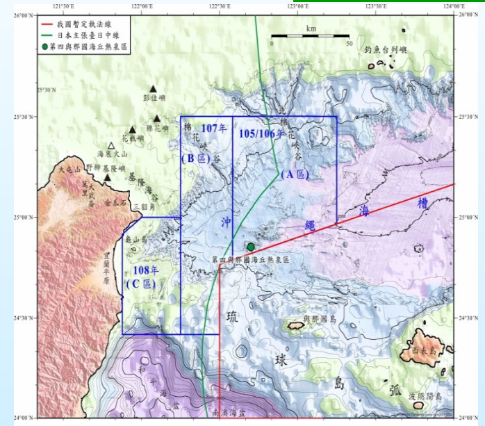
分年擇區調查
