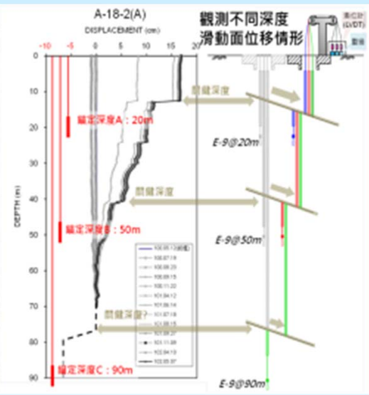
觀測技術研發應用
