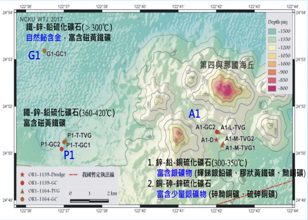
A1、P1及G1站位的金屬礦物種類
