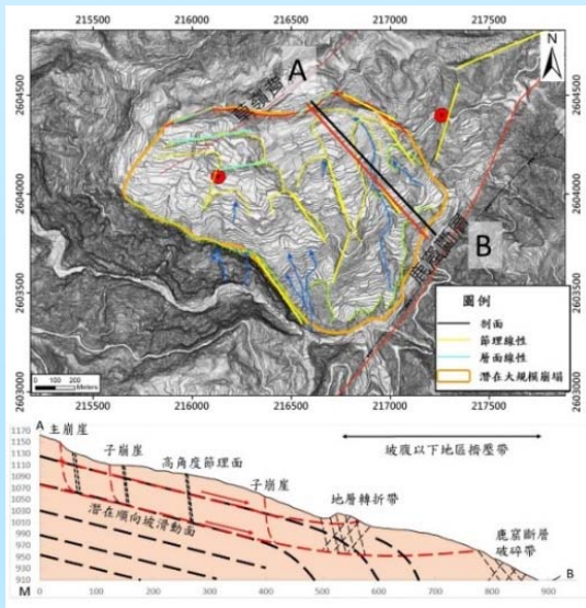
崩塌調查及判釋
