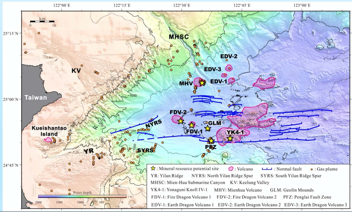
南沖繩海槽水深地形、主要正斷層(藍線)及6處礦產賦存潛能區(黃色星號)
