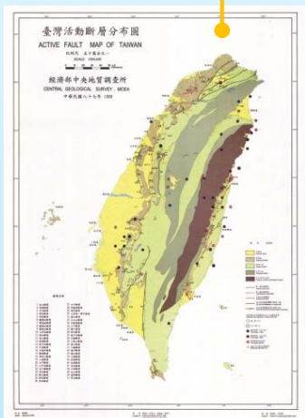
活動斷層分布圖第一版
