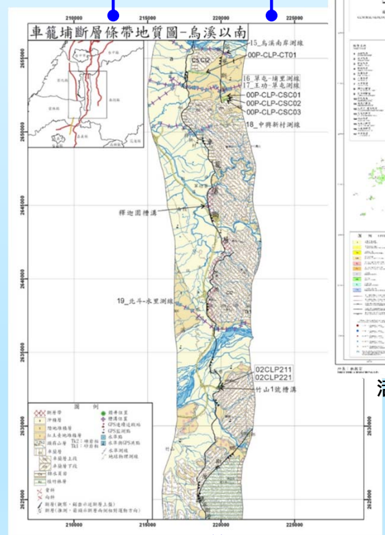
活動斷層條帶地質圖及說明書
