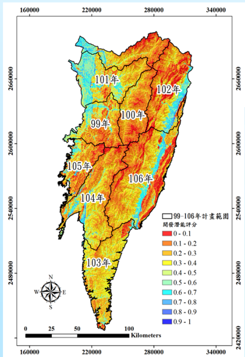
中段與南段山區地下水 開發潛能圖
