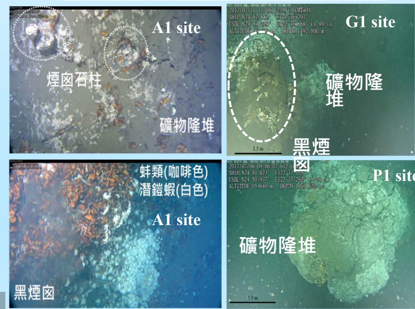
煙囪石柱、礦物隆堆及特有生物群落
