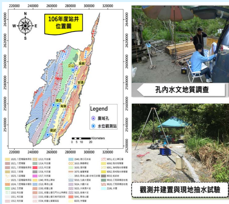
山區地下水觀測站網建置及 現地水文地質調查
