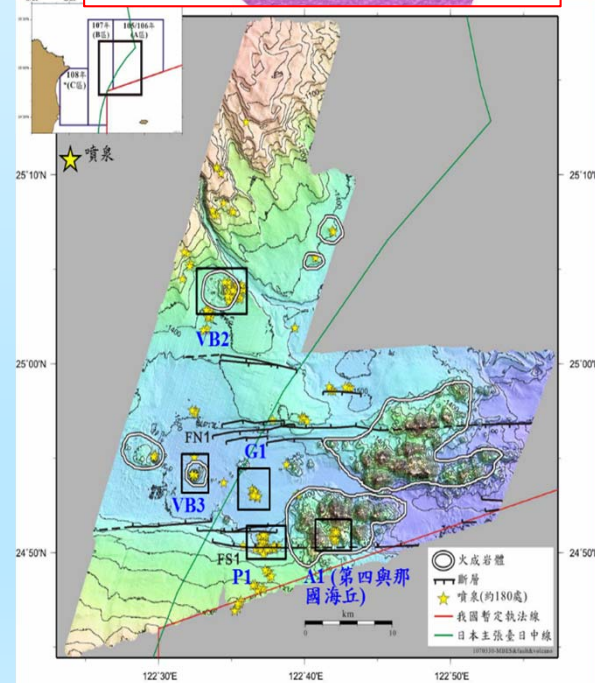
5處礦產資源潛能區分布圖
