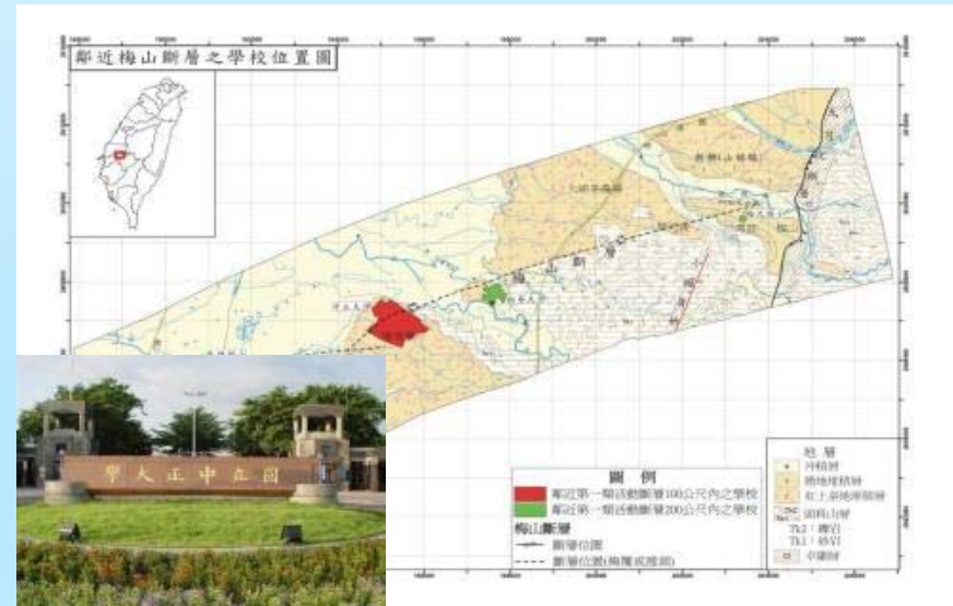
活動斷層調查及觀測
