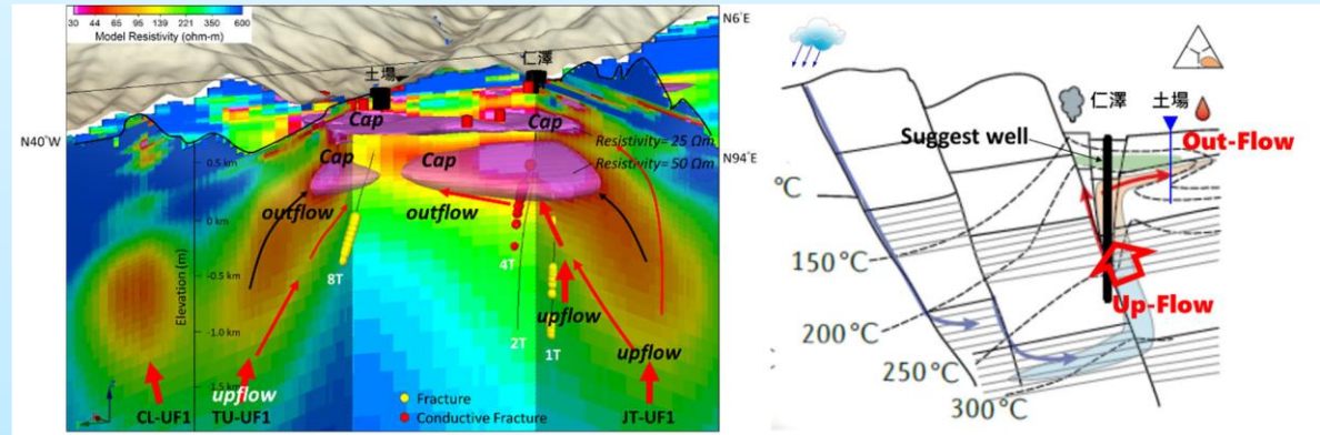
仁澤土場地熱概念模式
