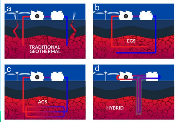
地熱發電種類 a. 傳統型地熱 b. 增強型地熱 c. 進階型地熱 d. 綜合型地熱
