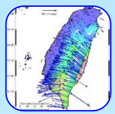
GPS 速度場
