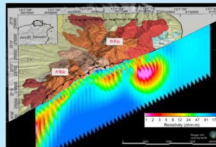
大屯山地區大地電磁地電阻剖面立體展示
