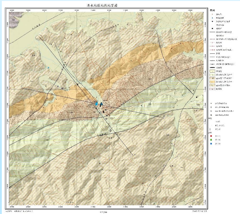
宜蘭清水地區地熱地質圖
