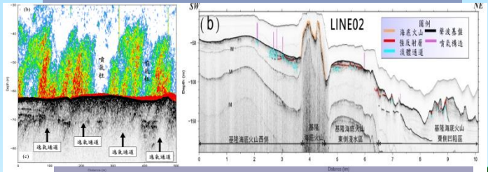
基隆海底火山有活躍噴氣活動
